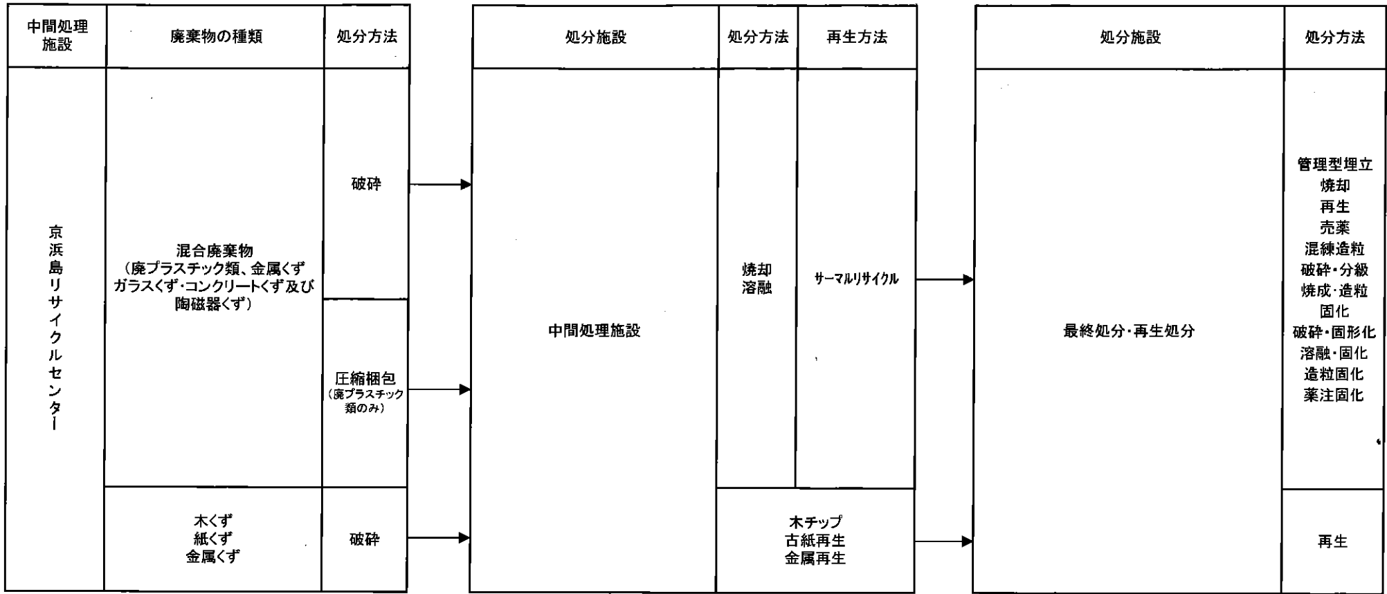
事業場ごとの産業廃棄物の処理工程図
